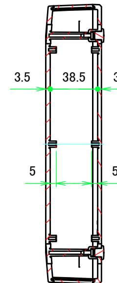
A-A ( 1 : 3 )
